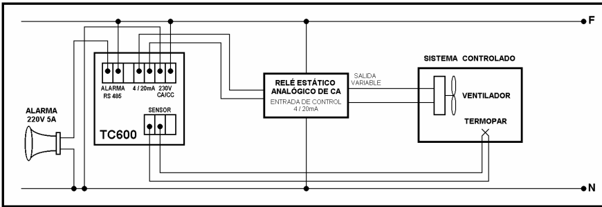
Ejemplo 3 Control de Salida Analógico (4 - 20mA) para un Relé Estático Analógico de CA. Control de Alarma por Relé Electromecánico. Señal de Entrada proveniente de un Termopar.
