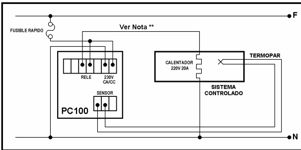
Ejemplo 1: Controlador con Salida de Relé sin conectar la Alarma
