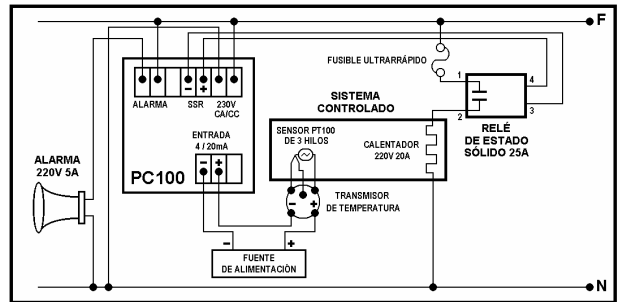
Ejemplo 2: Controlador con Salida de Relé de Estado Sólido (SSR) y Salida de Relé para la Alarma
