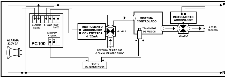
Ejemplo 3: Control de Salida Analógico (4 - 20mA) para una válvula. Control de Alarma por Relé. Señal de Entrada Analógica (4 - 20mA) de un transmisor de presión.
